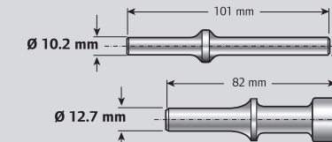
Jackset blank
